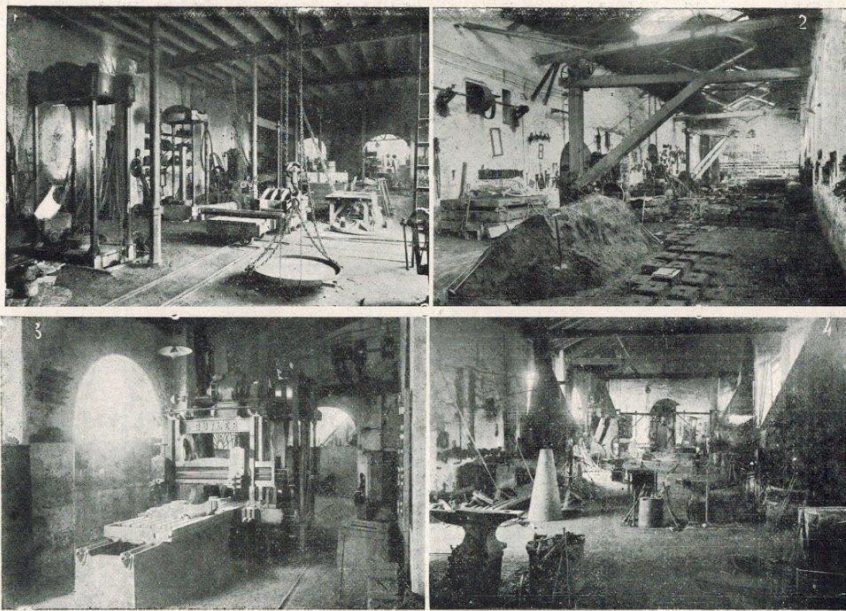
1. Taller de montaje de prensas y molinos para aceite. 2. Taller de fundición. 3. Máquina de cepillar de 3,00 m. X 1,25 m. X 1,25 m. 4. Taller de forja con su martillo pilón eléctrico de 5 quintales.
