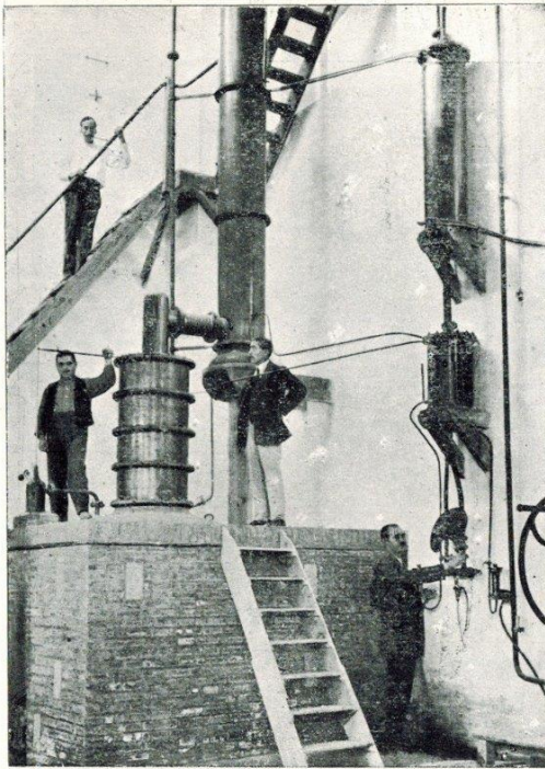
NOTABLE APARATO DESTILADOR DE ALCOHOL, DEL ACAUDALADO INDUSTRIAL D. E. FLORES MOLÍNS Dicho alambique, sin condensadores de agua, produce directamente el alcohol de 96° centesimales.
